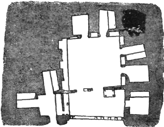
Fig. 8. Bhājā, Small Vihāra : Plan
